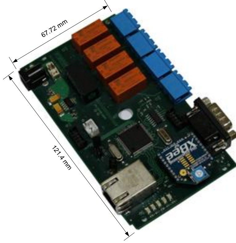
Şekil 1. UZAKRÖLE™ ET100Ethernet Mekanik Özellikleri
