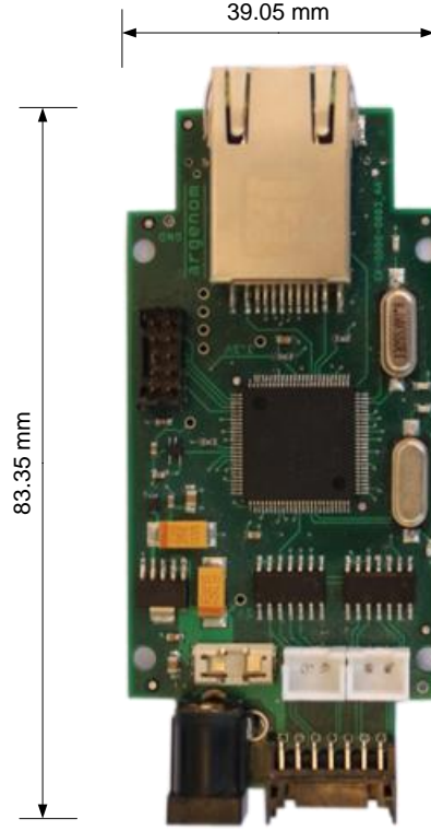
Şekil 1. Elektroduyu™ SN100Ethernet Mekanik Özellikleri
